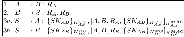
Fig. 1. 3PKD protocol
